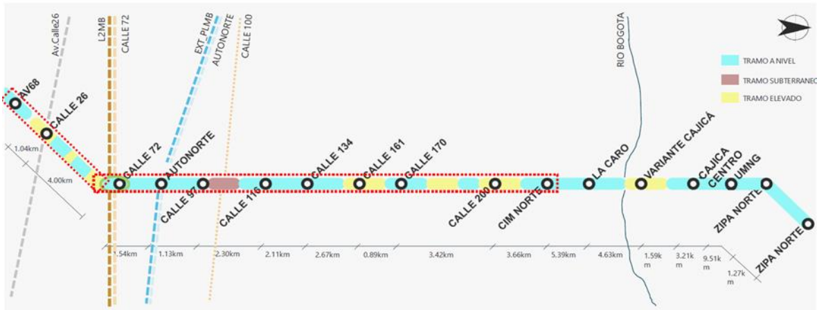
Ilustración 12 Trazado Regiotram Norte
