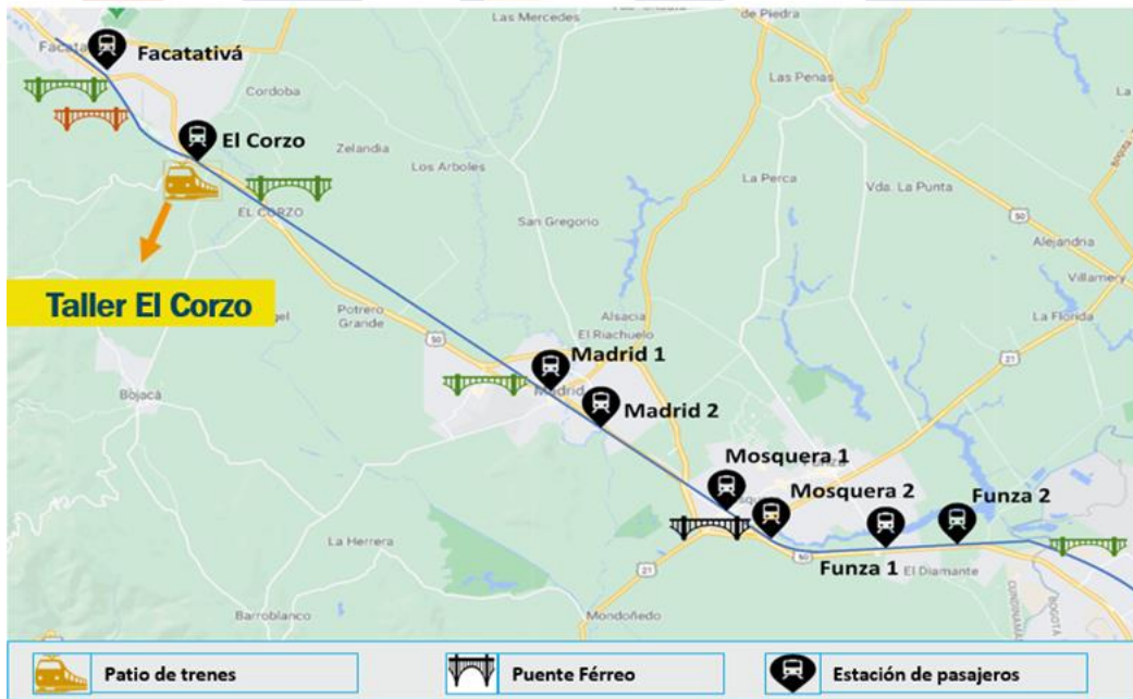
Ilustración 1. Trazado Sabana de Occidente
